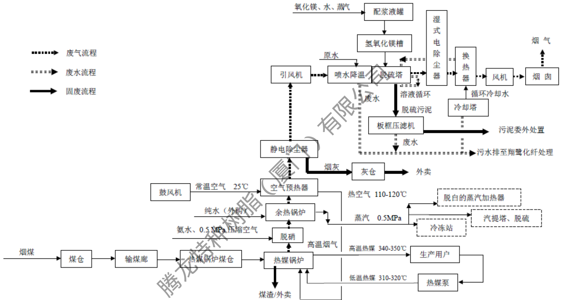
图 2.4-5 公用课热媒锅炉生产过程工艺流程和产污环节示意图
