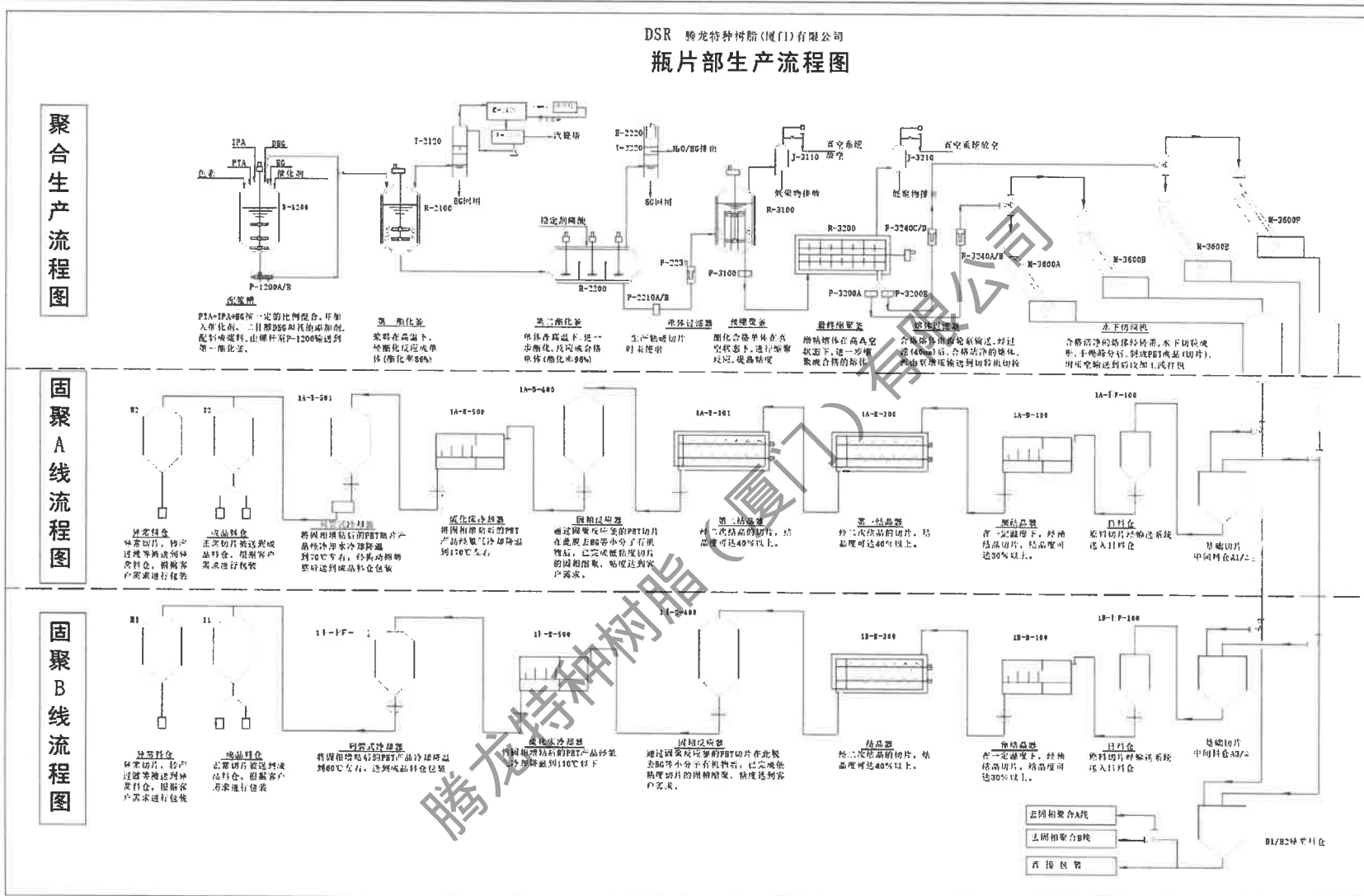
图 2.4-3 瓶片部生产流程总图
